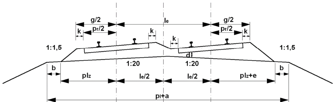
Slika 11: Prečni presek tirne grede dvotirne proge v krivini
