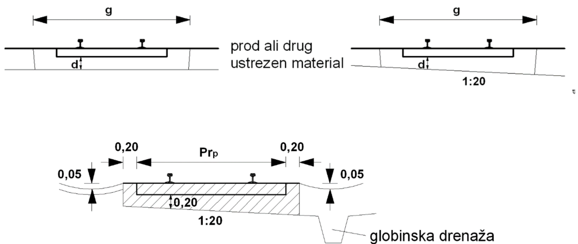
Slika 13: Prečni prerez tirne grede na postajnih in industrijskih tirih
