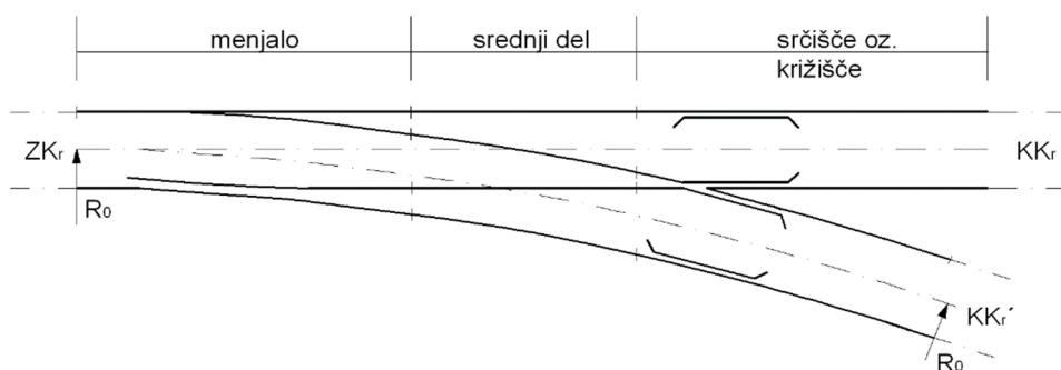
Slika 15: Enojna kretnica
