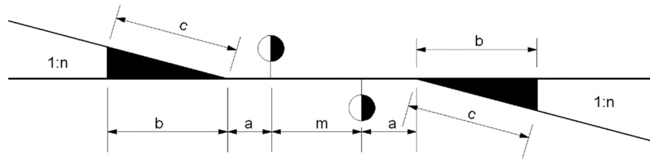
Slika 18: Vmesna prema med kretnicama
