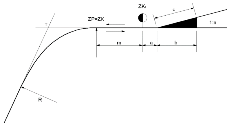
Slika 21: Vmesna prema med kretnico
