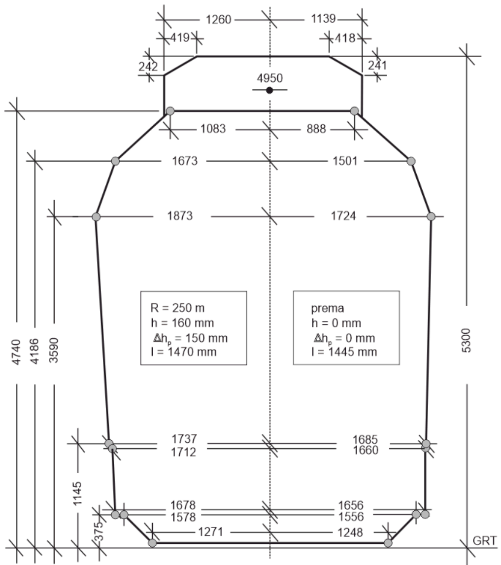
Slika 3: Minimalni svetli profil DE3 za R \geq 250 m
