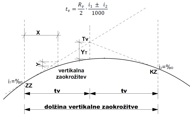
Slika 2: Vertikalna zaokrožitev
