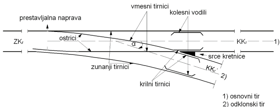
Slika 16: Sestavni deli enojne kretnice
