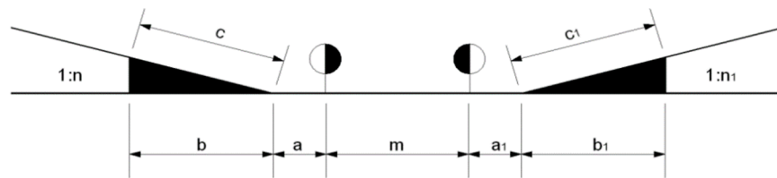
Slika 19: Vmesna prema med kretnicama
