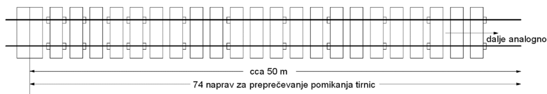
Slika 23: Vgradnja naprav za preprečevanje vzdolžnega pomika tirnic 49 E
