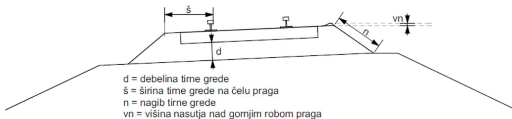
Slika 14: Prečni presek tirne grede
