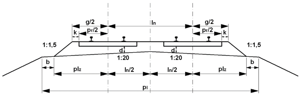
Slika 9: Prečni presek tirne grede v krivini in enostranskem nagibu planuma
