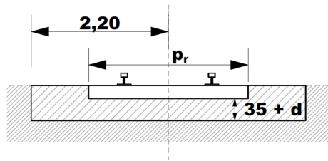
Slika 12: Tirna greda v območju umetnih objektov
