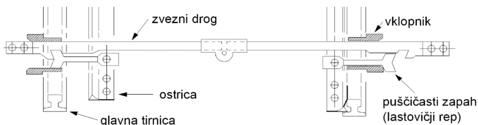
Slika 17: Puščičasti kretniški zapah
