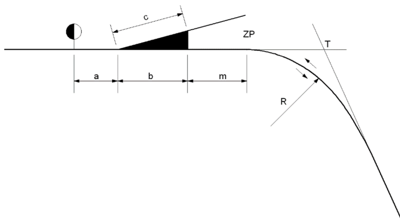
Slika 22: Vmesna prema za kretnico
