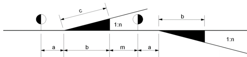
Slika 20: Vmesna prema med kretnicama
